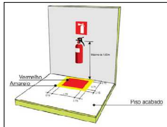
Figura 16: Detalhe de instalação de extintores em áreas sujeitas à Obstrução
