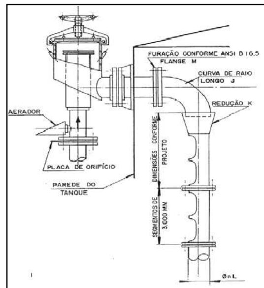
Figura 23: Sistema fixo de espuma
