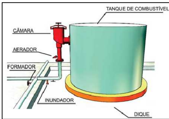
Figura 25: Detalhe de câmara de espuma
