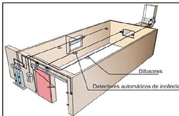
Figura 26: Sistema de CO 2
