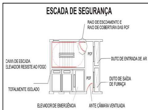
Figura 15: Escada e elevador à prova de fumaça
