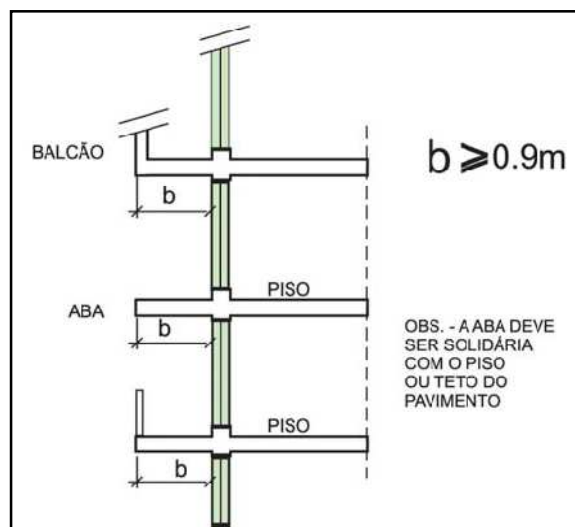
Figura 12: Compartimentação por aba horizontal ou balcão
