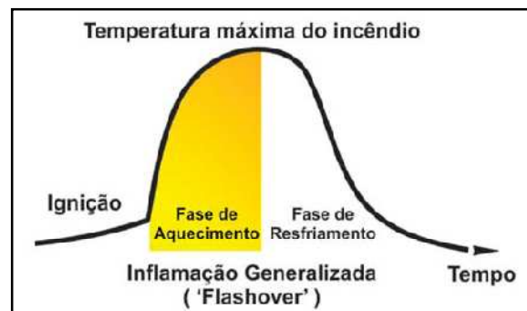
Figura 03: Curva temperatura - tempo de um incêndio
