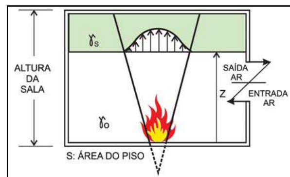
Figura 06: Processo de formação de gases e fluxo básico do ar
