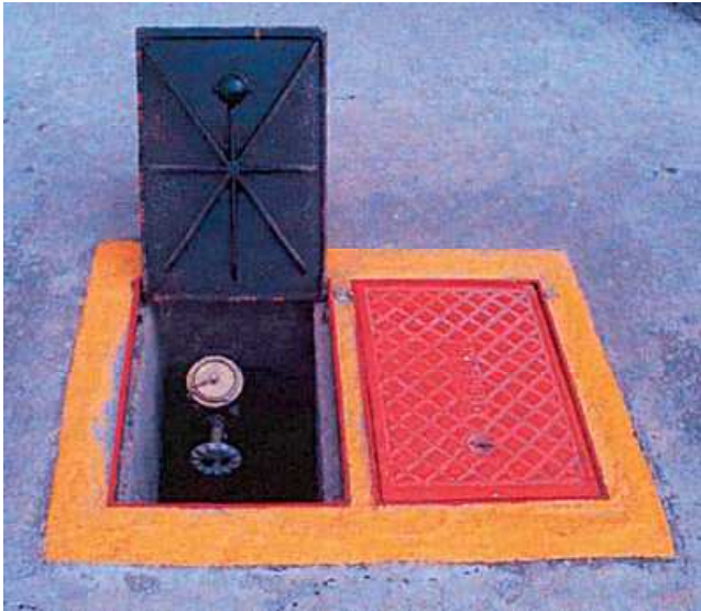
Figura 18: Registro de recalque para bombeiros
