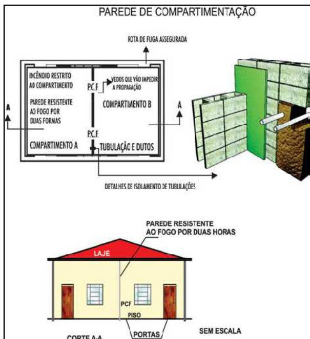
Figura 10: Detalhes de parede de compartimentação
