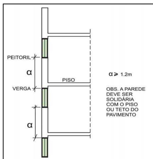
Figura 11: Distância de afastamento entre verga e peitoril
