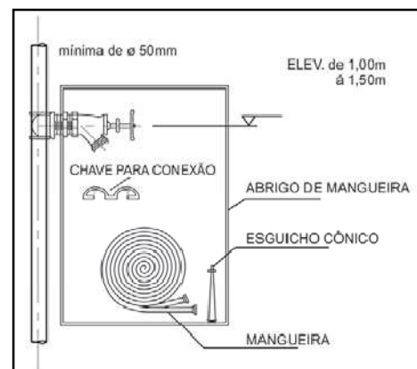
Figura 17: Detalhe de hidrante
