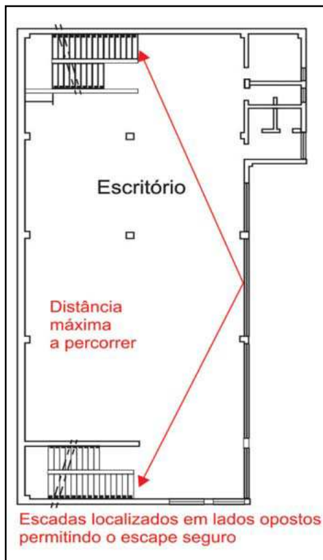
Figura 14: Localização e caminhamento para acesso a uma escada
