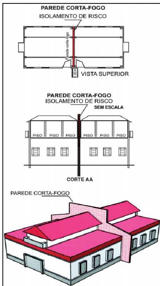
Figura 09: Isolamento obtido por parede corta-fogo
