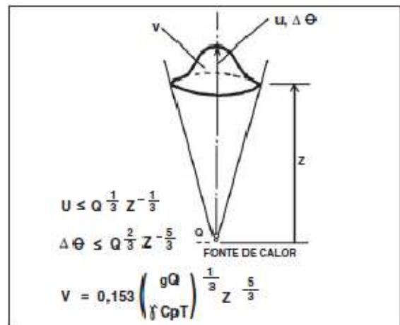
Figura 05: Plume de fumaça
