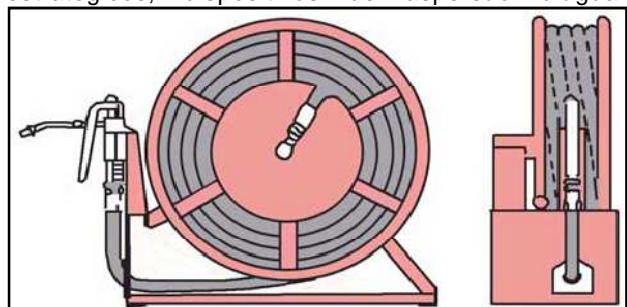
Figura 21: Sistema de mangotinhos
