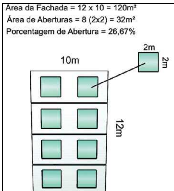
Figura 11: Porcentagem de aberturas na fachada
