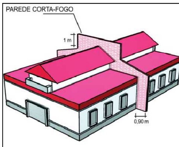
Figura 8: Parede corta-fogo
